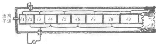
图61 直线加速器的原理
