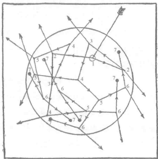
图 64 在一块球形裂变物质中由一个中子引发了核链式反应。虽然许多中子会穿过表面离开，但连续几代的中子数量仍在增加，最终导致爆炸
