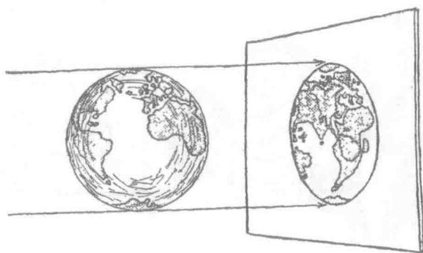
图20 地球的平面投影
