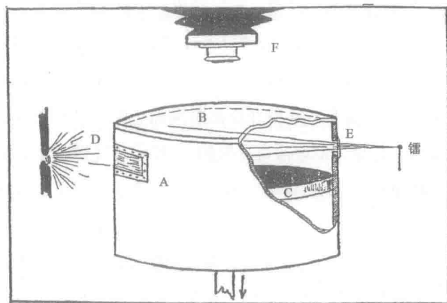
图58 威尔逊云雾室图解
