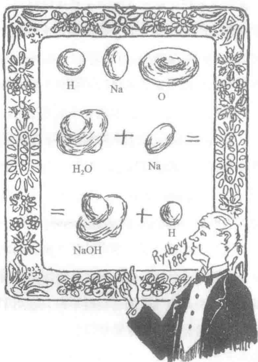
图39 里德伯 (Rydberg), 1885
