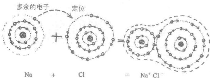
图42 氯化钠分子中钠原子和氯原子结合的示意图
